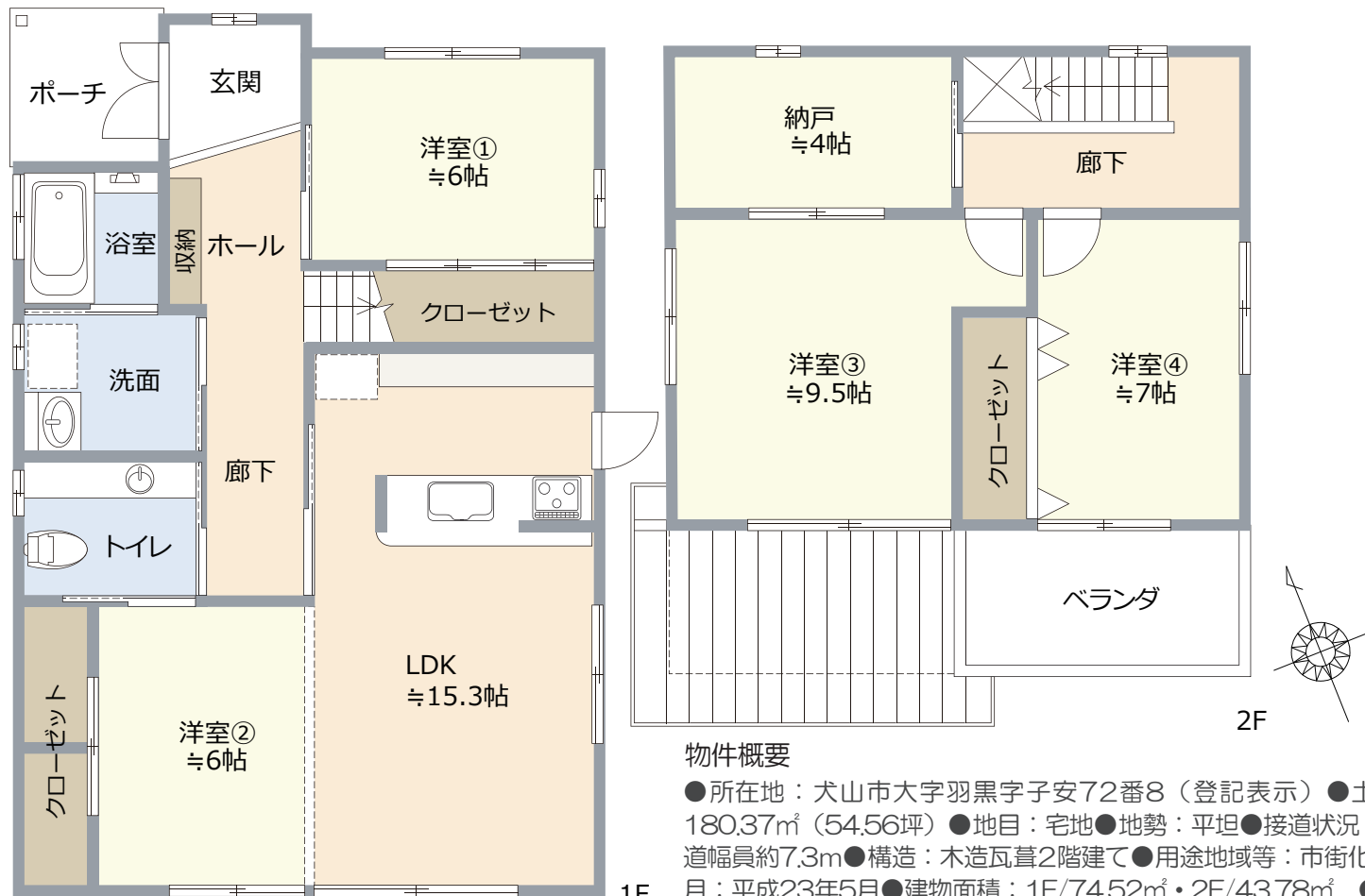
間取図
