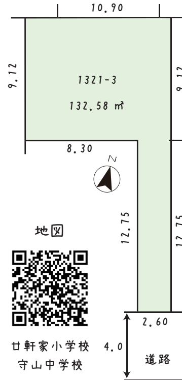
敷地配置図
