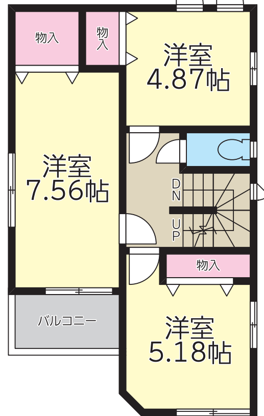
2階平面図:42.08㎡(12.72坪)
