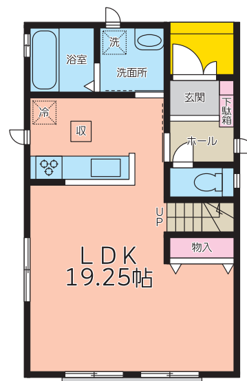
1階平面図:47.21㎡(14.28坪)
