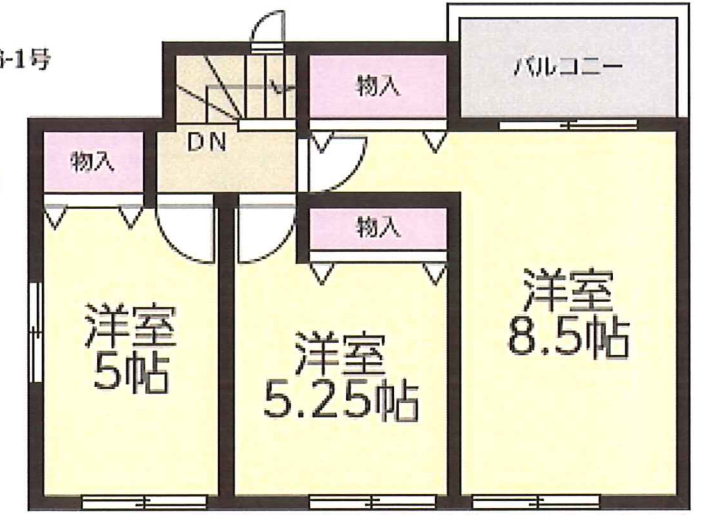
3階平面図:38.30㎡(11.58坪)
