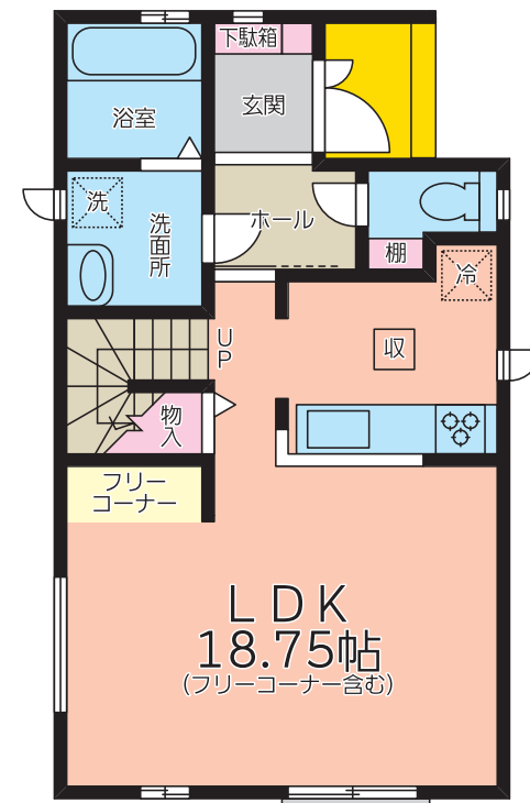
1階平面図:48.03㎡(14.52坪)
