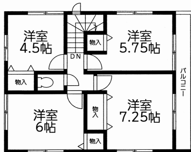
2階平面図:49.27㎡(14.90坪)
