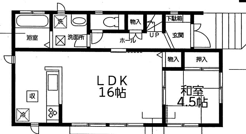
1階平面図:52.17㎡(15.78坪)
