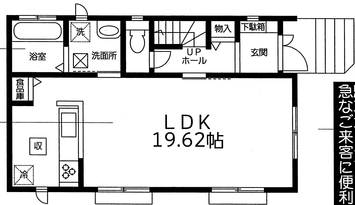
1階平面図:48.85㎡(14.77坪)
