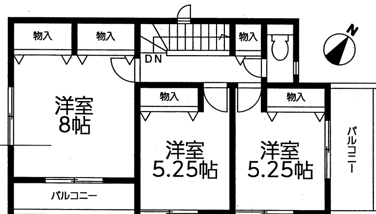
2階平面図:44.71㎡(13.52坪)
